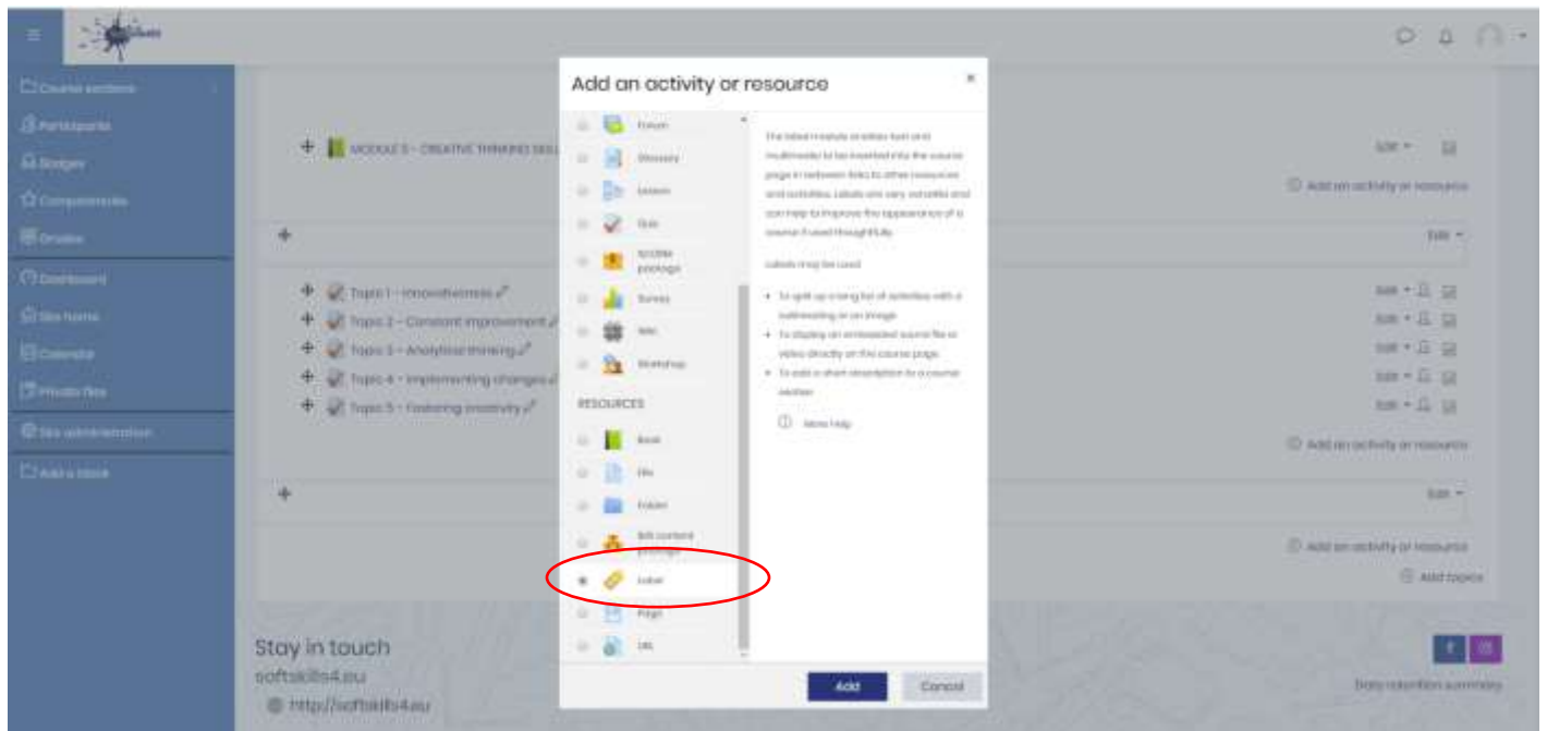
Slika 19: Dodavanje oznake
