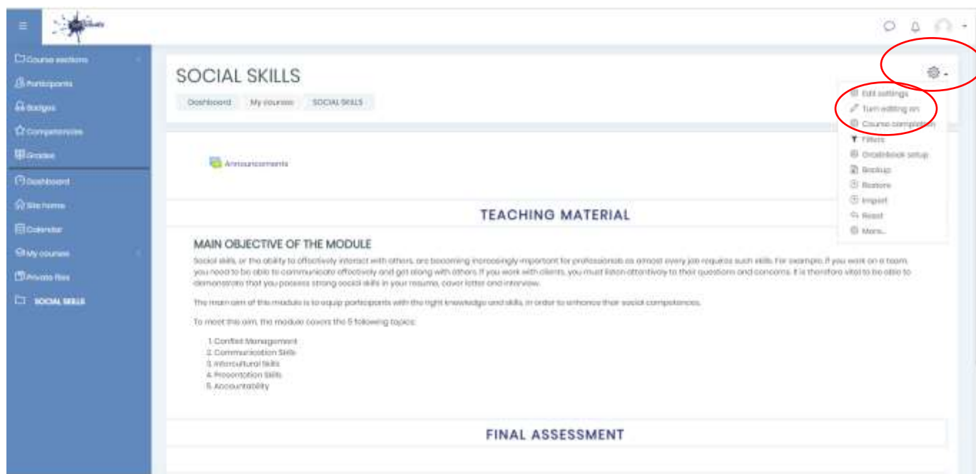
Slika 4: "Uključi uređivanje"
