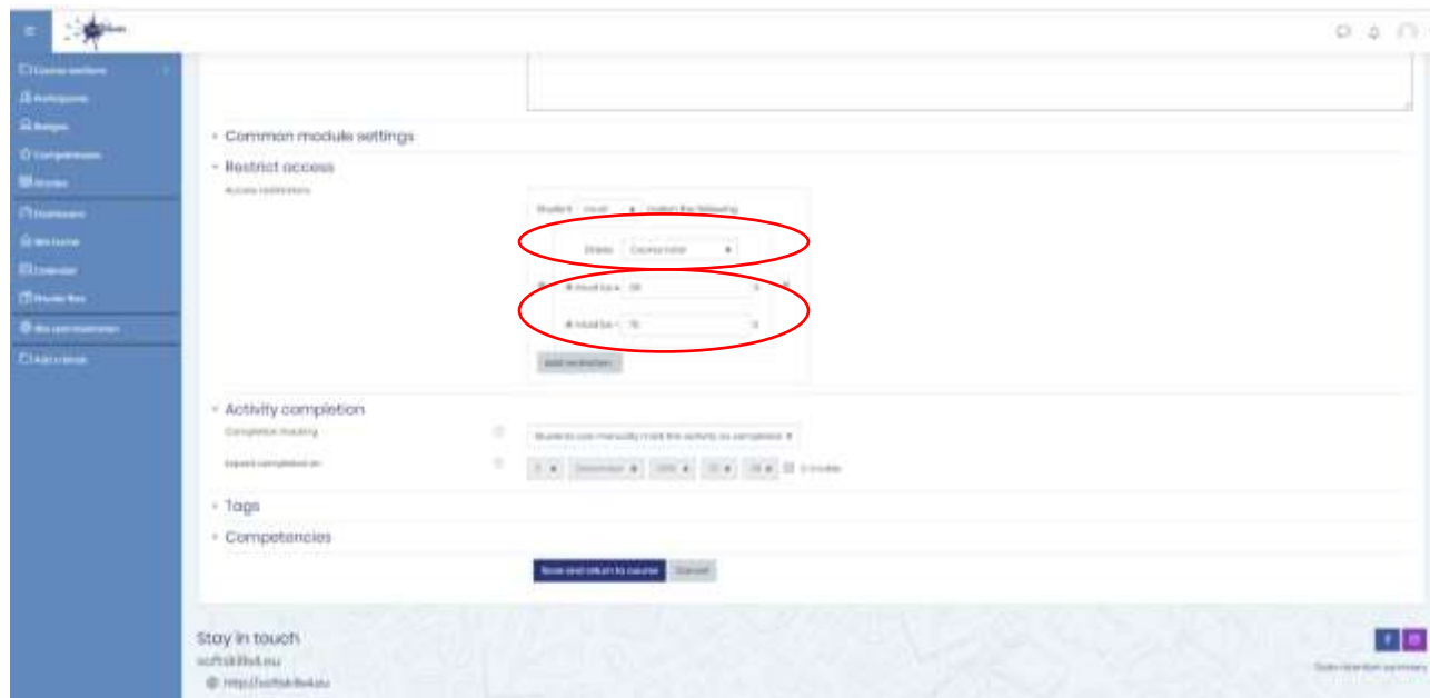
Slika 20: Postavke oznaka
