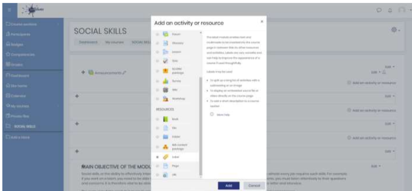
Slika 6: Dodajte oznaku
