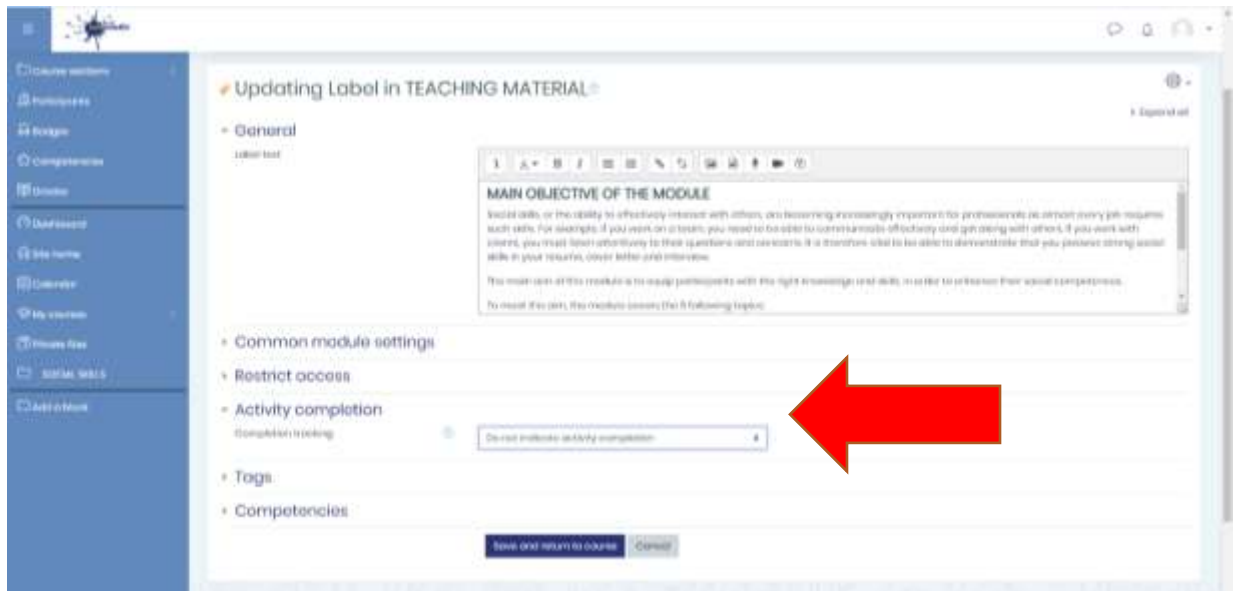
Slika 7: Završetak aktivnosti
