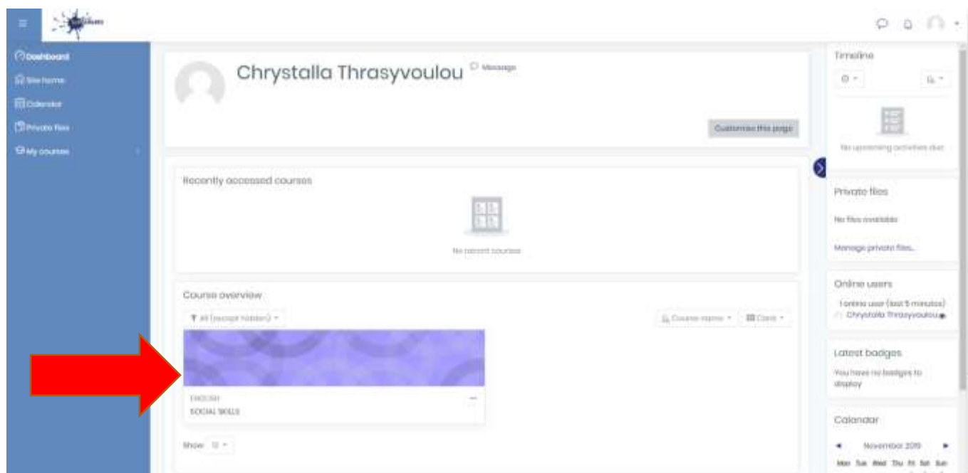
Slika 3: Modul
