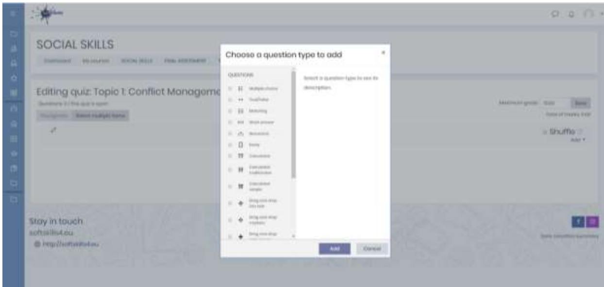
Slika 18: Vrste pitanja
