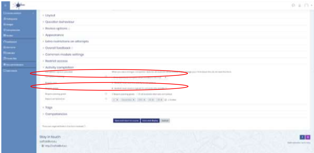
Slika 15: Postavke Kviza
